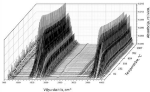
2. attēls. Termogravimetrija/diferenciāli termiskā analīze un izdalīto gāzveida vielu infrasarkanie spektri W nanoslānim uz Si-SiO 2 pamatnes.
