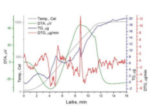
2. attēls. Termogravimetrija/diferenciāli termiskā analīze un izdalīto gāzveida vielu infrasarkanie spektri W nanoslānim uz Si-SiO 2 pamatnes.
